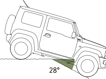
Overklimhoek voor
